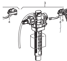
Vanne de remplissage Type 360
