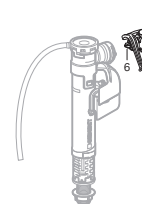
Vanne de remplissage Type 34x
