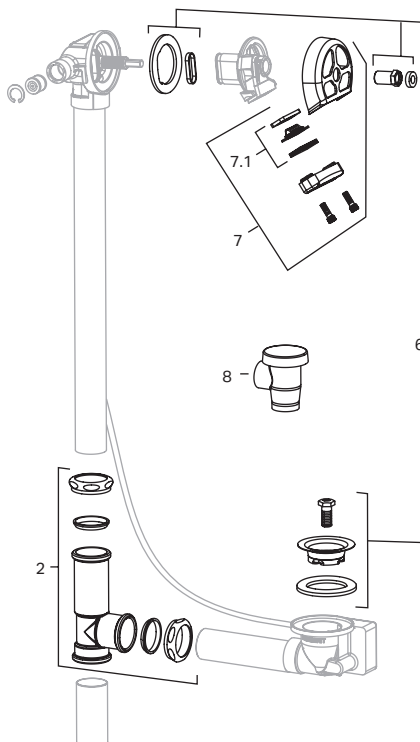
Remplisseuse de baignoire en cascade
