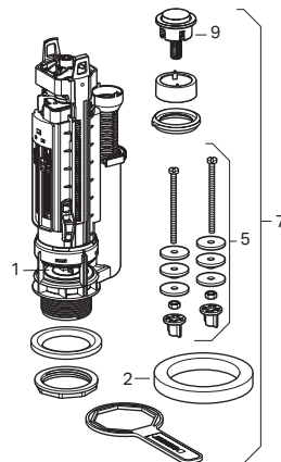
Vanne de remplissage Type 290, chasse simple
