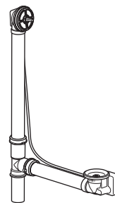
Fig. A Unité de robinetterie brute tubulaire
